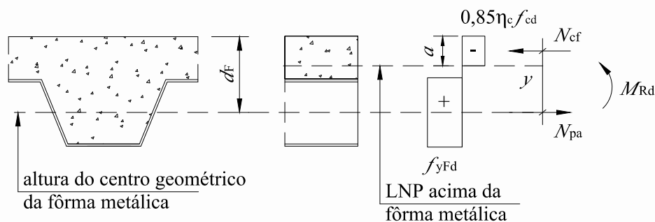
Figura N.2 – Diagrama de tensões para o momento positivo – Linha neutra plástica acima da fôrma de aço
