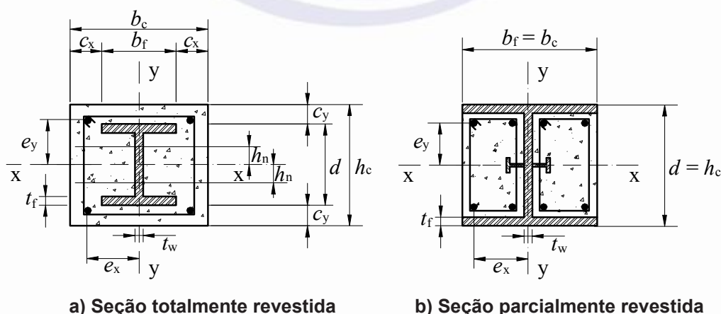
Figura M.6 – Seção revestida com concreto, fletida em relação ao eixo x
