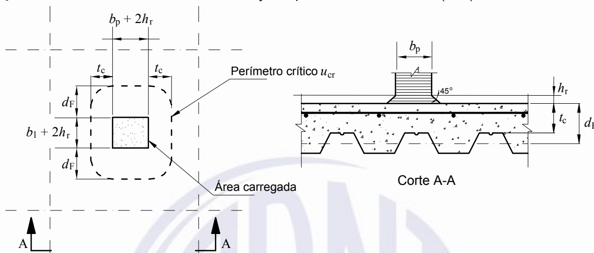
Figura N.6 – Perímetro crítico para punção
