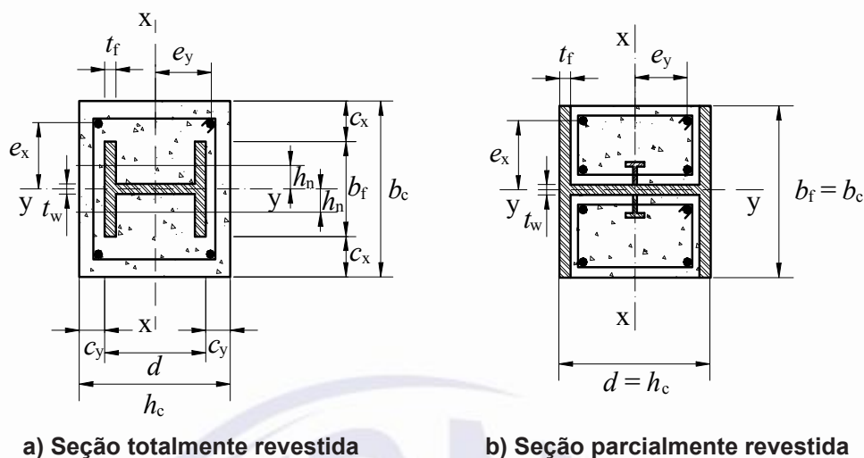
Figura M.7 – Seção revestida com concreto, fletida em relação ao eixo y
